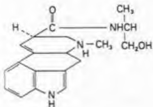
ERGONOVINE
